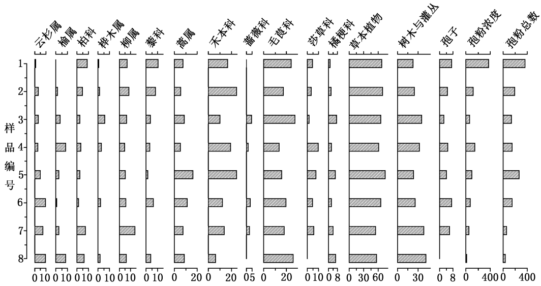
图七 第8层Q区孢粉图谱
